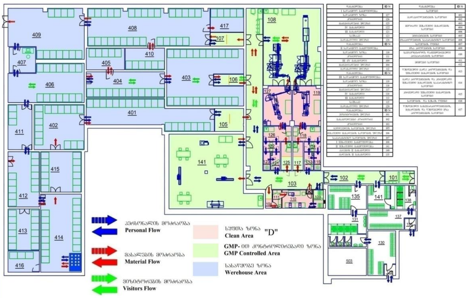
შპს "ავერსი-რაციონალი"-ს წარმოების და საწყობის სქემა მასალების და პერსონალის მიმოქცევაში Lay out of production and storage areas of "Aversi-Rational" including the material and personnel flows
